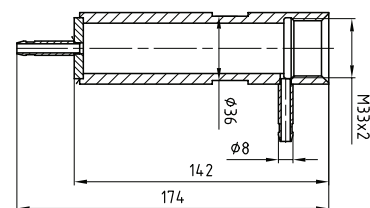
кювета ВР 69.10.270-01
