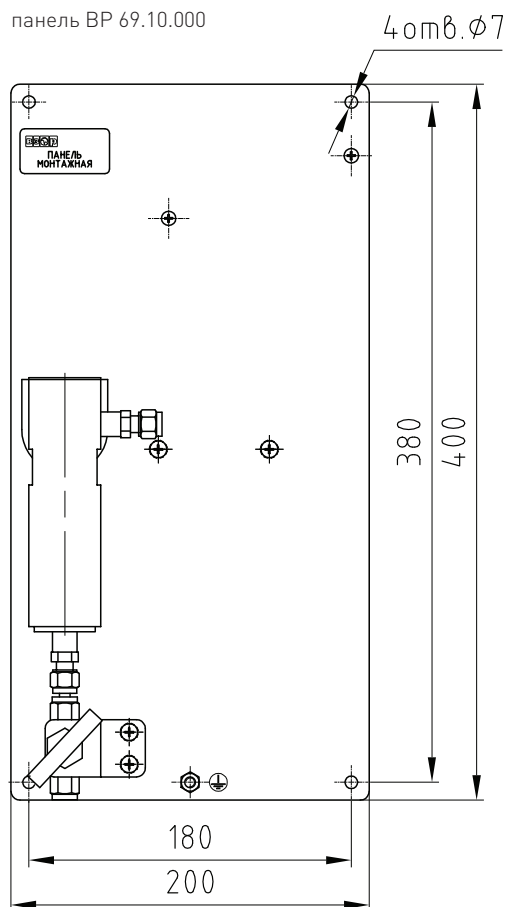
панель ВР 69.10.000
